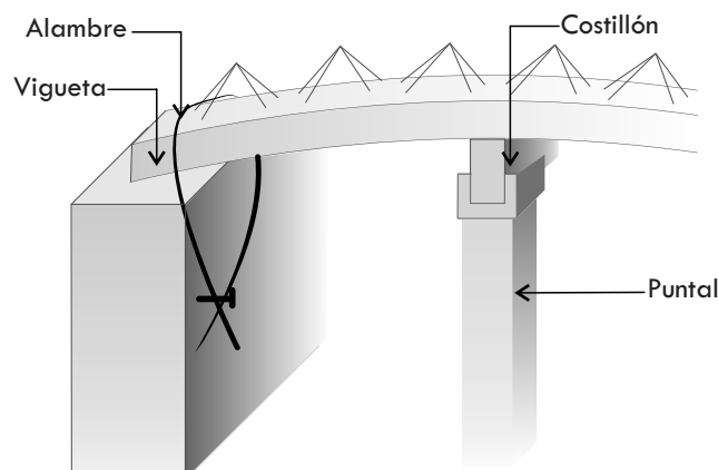
Figura 2 – Contraflecha Detalle de resolución
